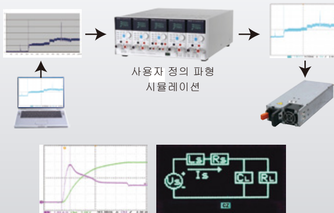
일정한 임피던스 모드 (CZ Mode)
